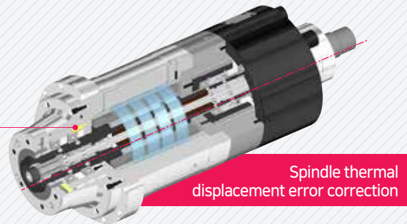
Thermal Sensor
